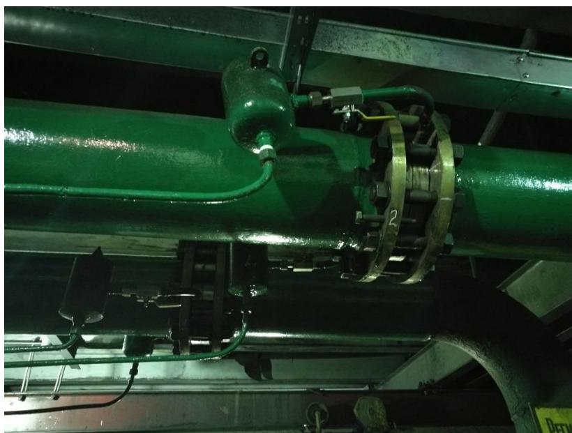
Расходомерные устройства котлов КВТС №1 и №2
