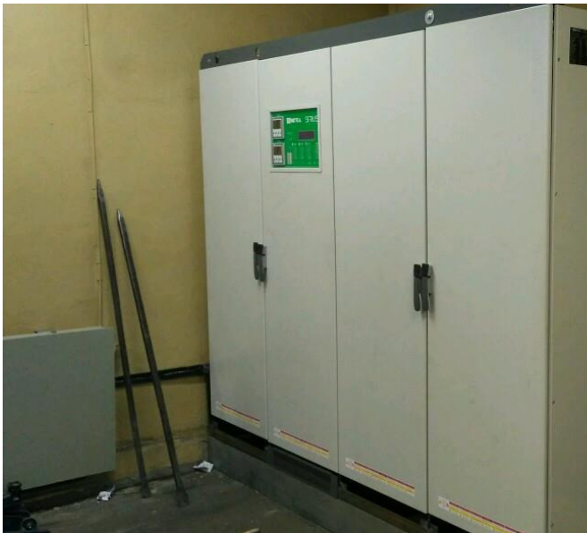
Стабилизатор напряжения Sirius 1000-15
