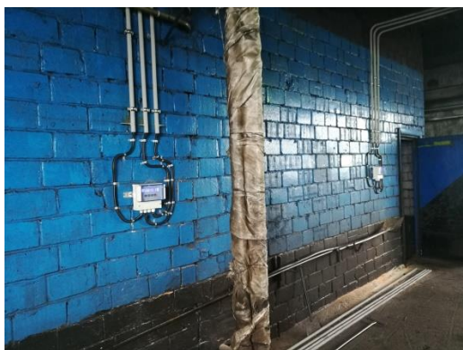
Монтаж конвейерны х весов
