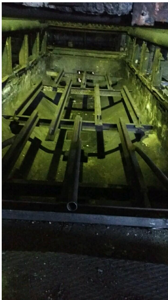
Монтаж щек топки Котла №2 КВТС-30
